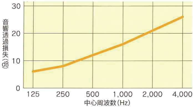
サウンドシャッター音響透過損失
