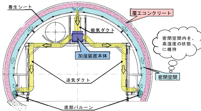
正面図
