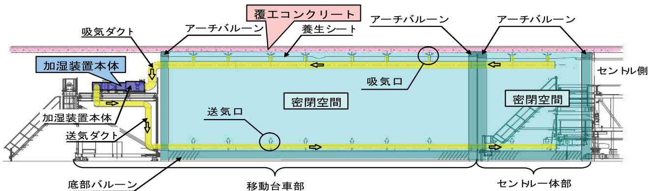
側面図
