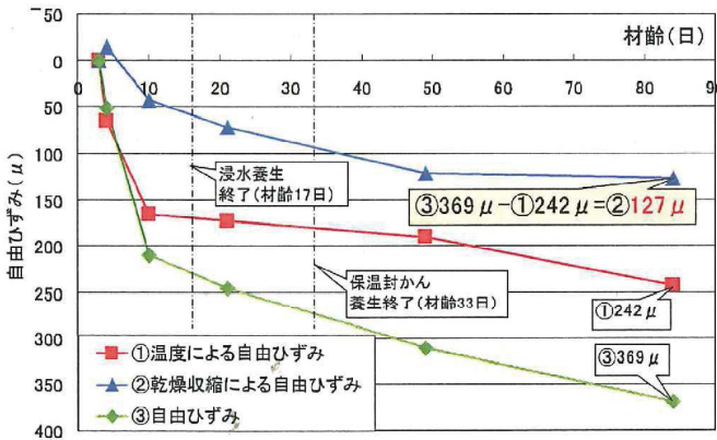
図-3 封かん養生
