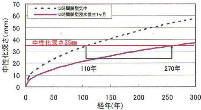
図-1 中性化促進
