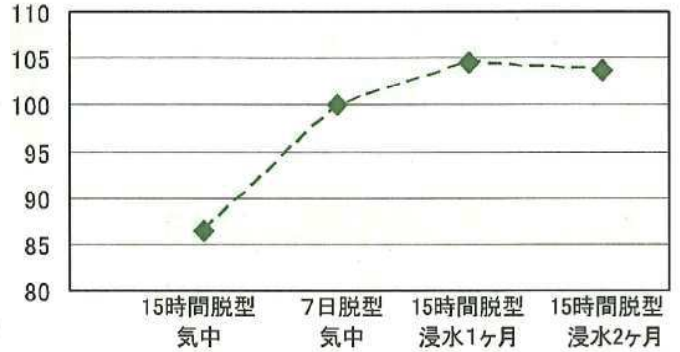
図-2 圧縮強度比較
