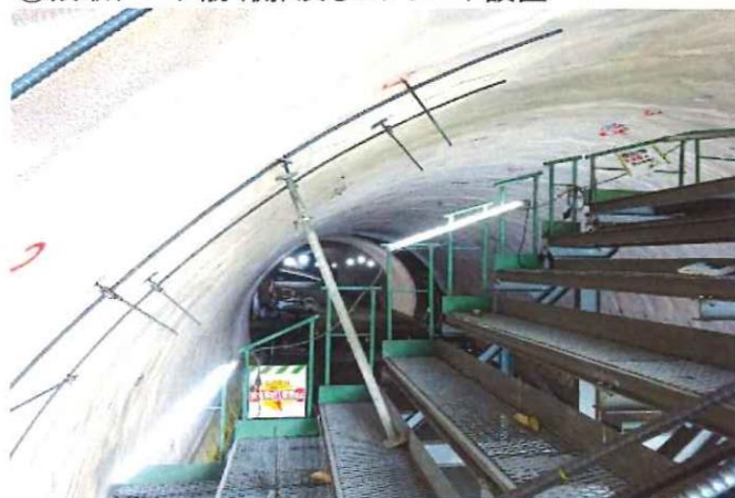
④段取アーチ筋組立終了⇒主筋・配力筋組立
