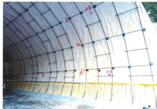
④段取アーチ筋組立終了⇒主筋・配力筋組立
