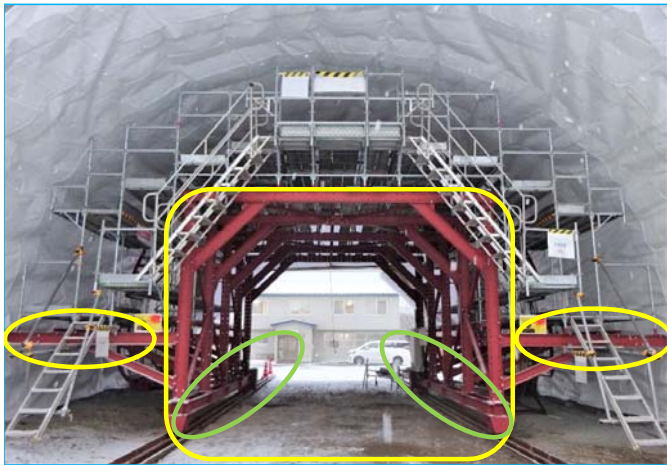
写真-1 黄色○部:基礎部材 緑色○部:駆動部
